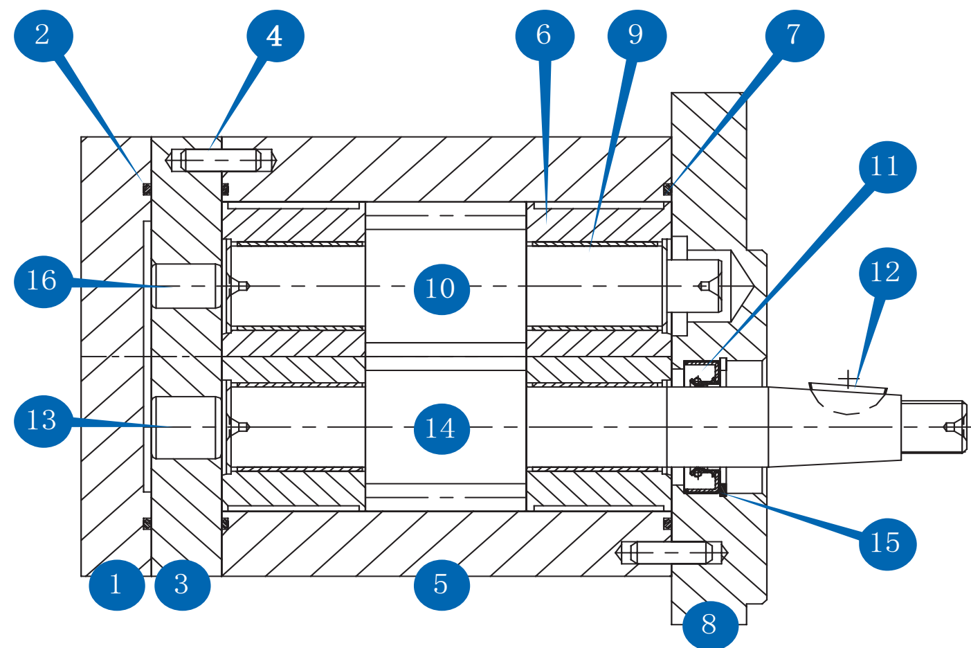
航空航天地面试验台液压泵分解图
