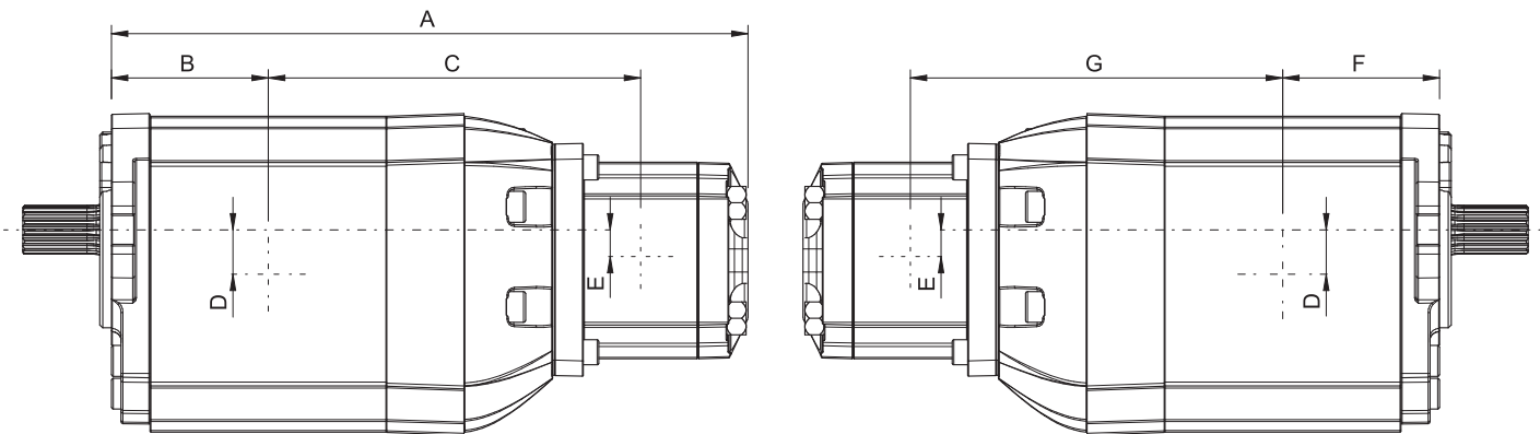
YT55+TD28双联液压泵参数表及尺寸图
