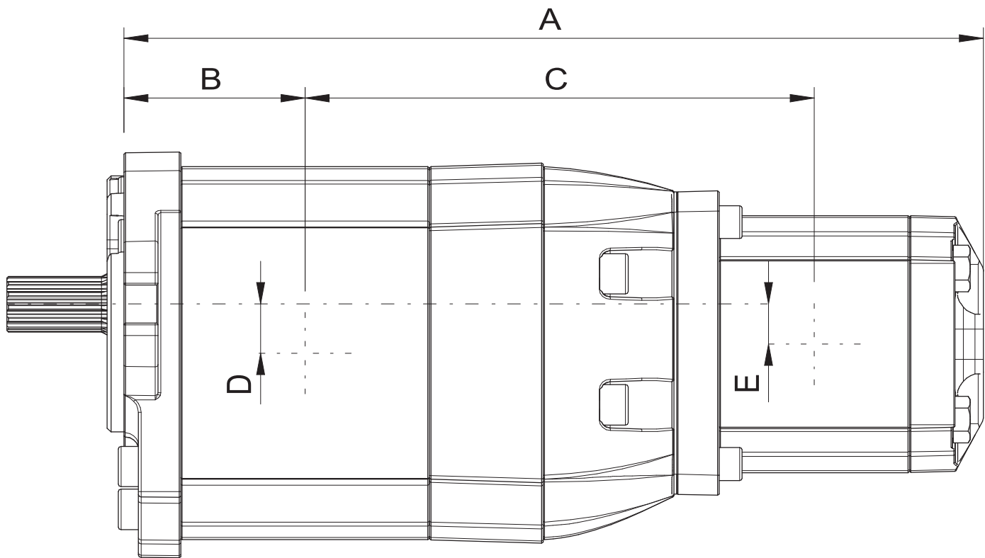
RA47+TD28双联液压泵参数表及尺寸图
