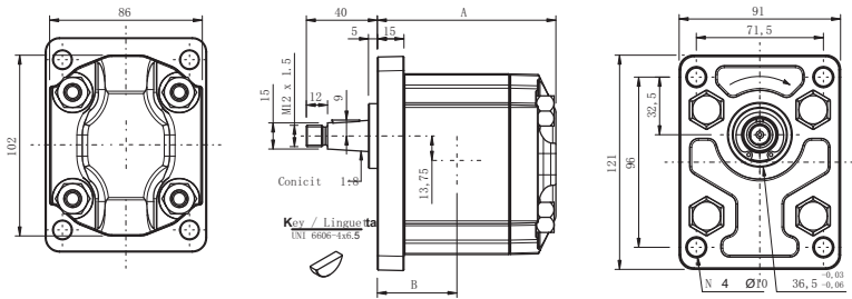
连接形式: 2-C4
