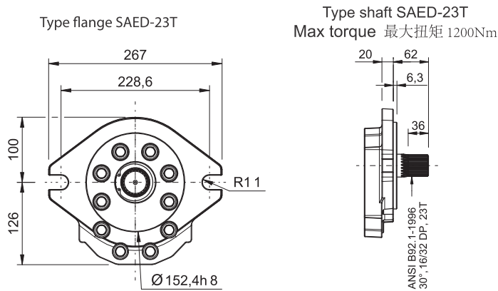
MD72系列可用的法兰和轴
