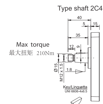
ZF38系列可用的法兰和轴
