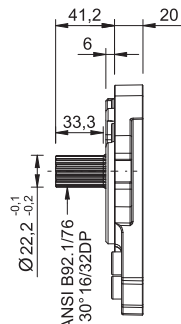
Type shaft SAEB-T13 Max torque 最大扭矩 600Nm
