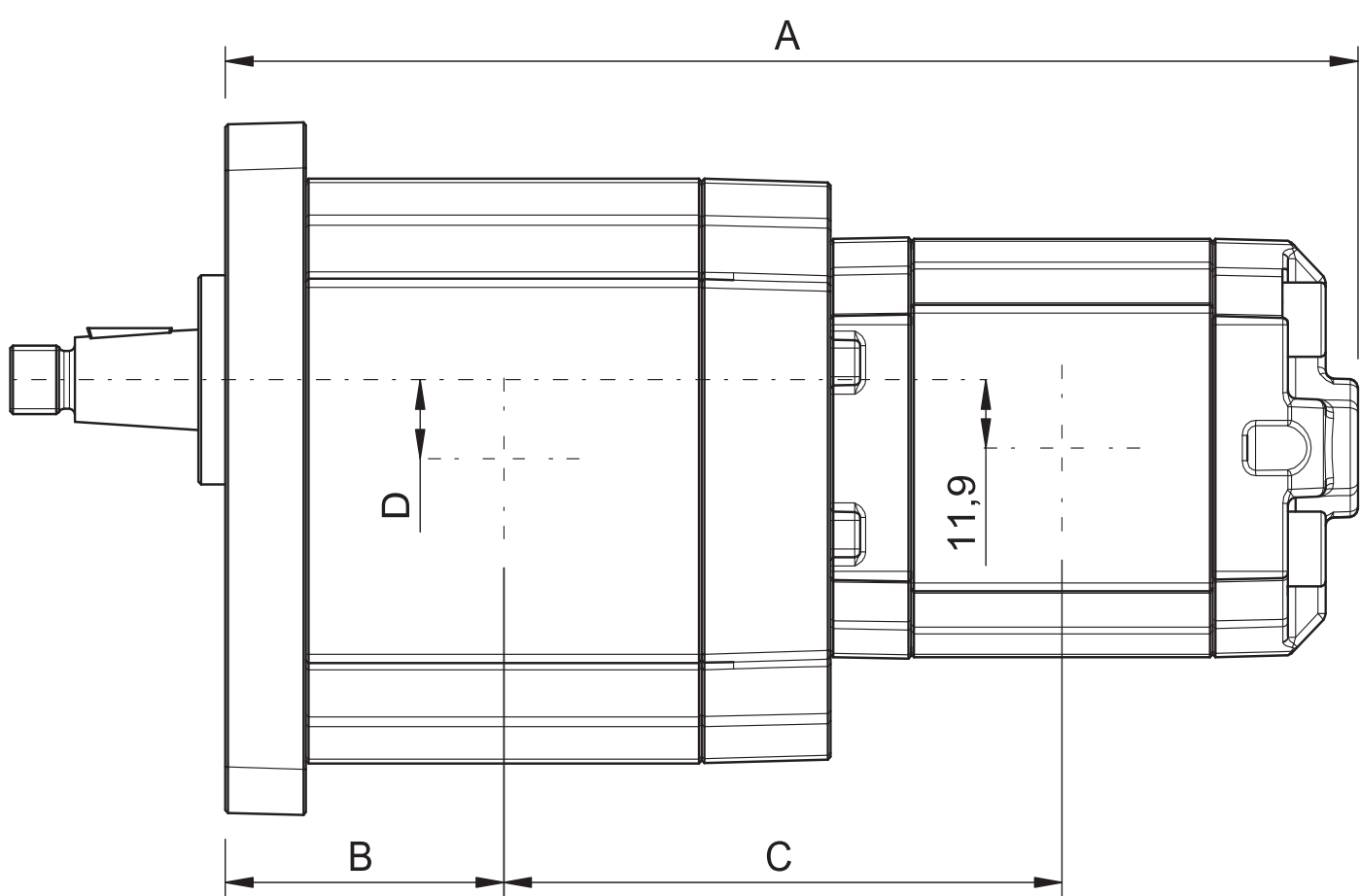
PD33+TD28双联液压泵参数表及尺寸图
