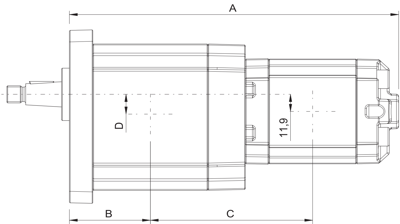
ZF38+TD28双联液压泵参数表及尺寸图
