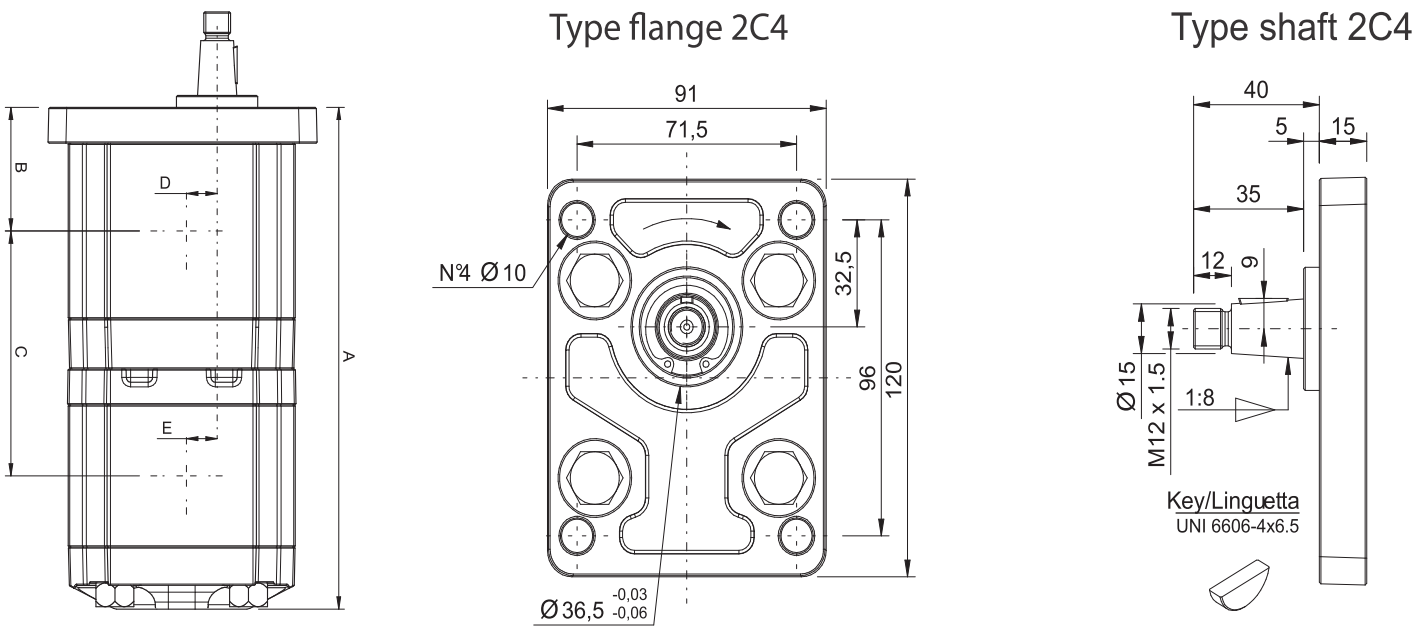
PD33+PD33双联液压泵参数表及尺寸图
