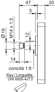
Type shaft 3-C9 Max torque 最大扭矩 320Nm
