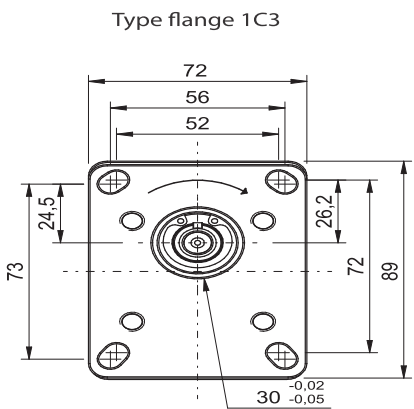
TD28系列可用的法兰和轴
