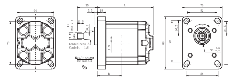
TD28系列安装尺寸表
