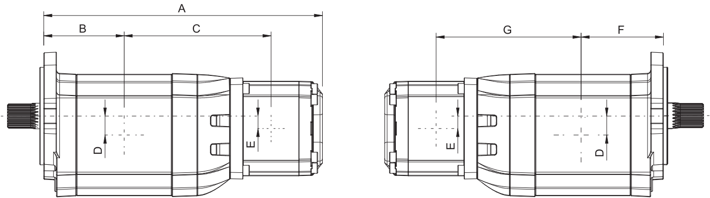
MD72+RA47双联液压泵参数表及尺寸图
