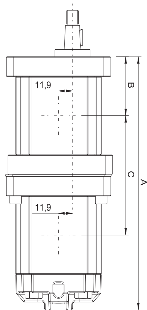
TD28+TD28双联液压泵参数表及尺寸图
