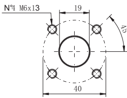
可选进出油口 Type Q
