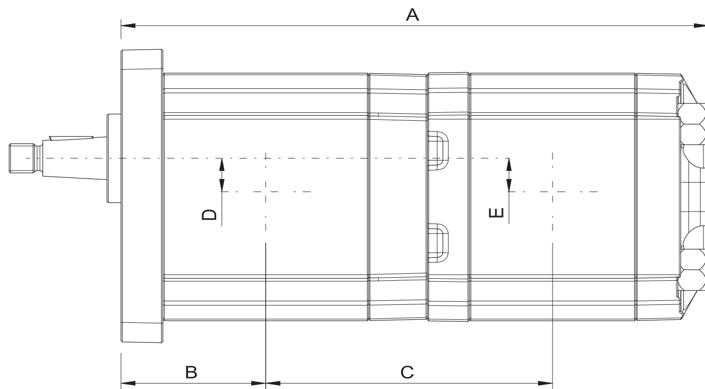
ZF38+PD33双联液压泵参数表及尺寸图
