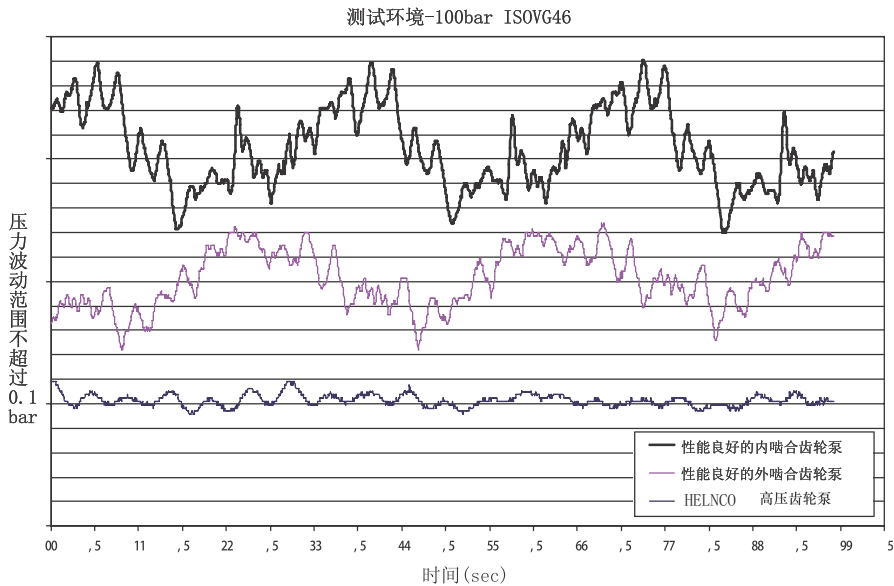
左图为实验室测试的各种高压泵工作状态下的压力波动范围
