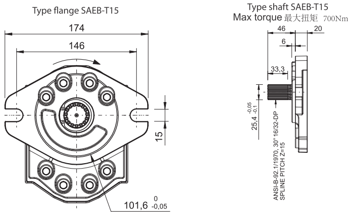
YT55系列可用的法兰和轴
